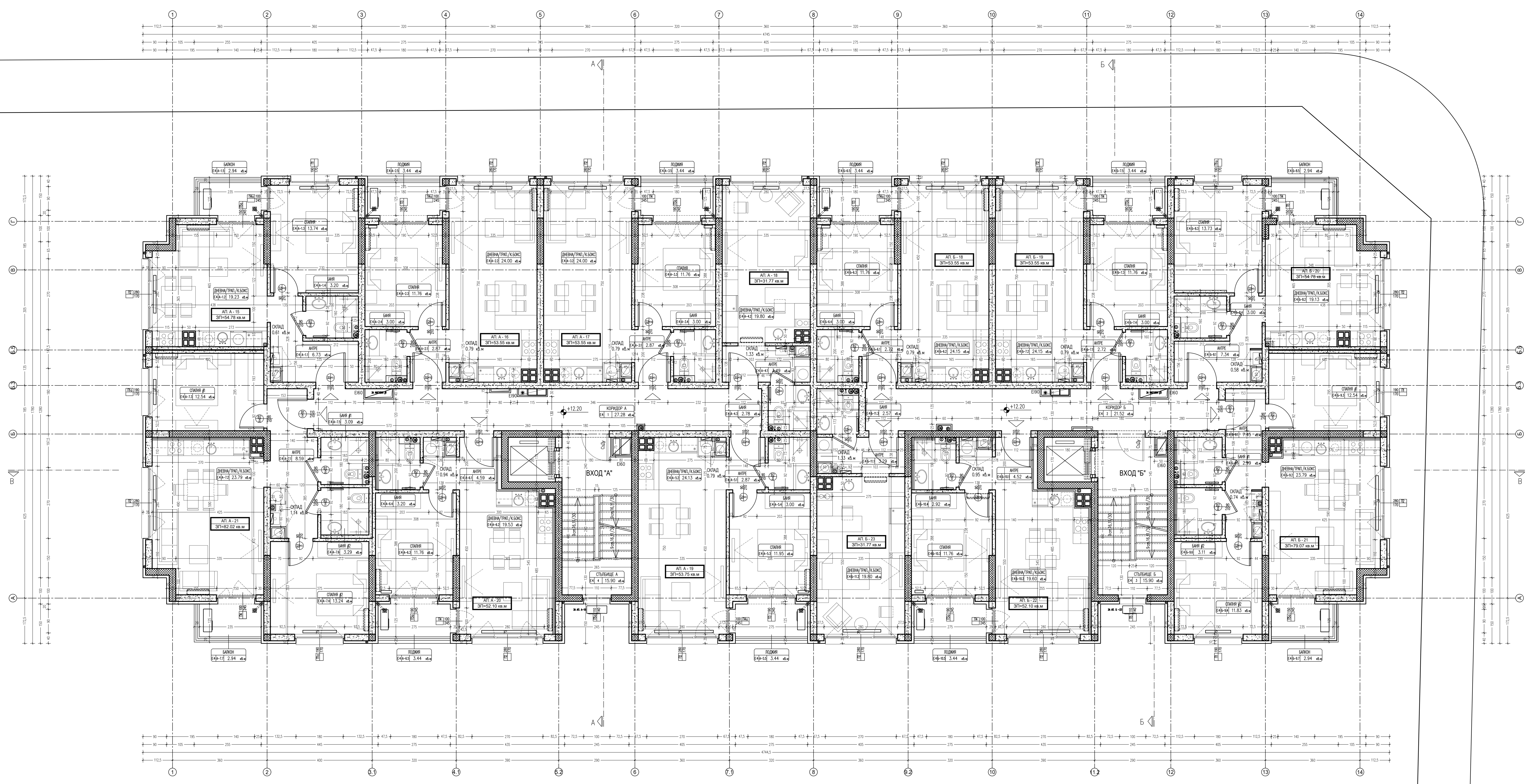
ПЛАН НА КОТА +12.20 / ЕТАЖ 4 / М 1:50
