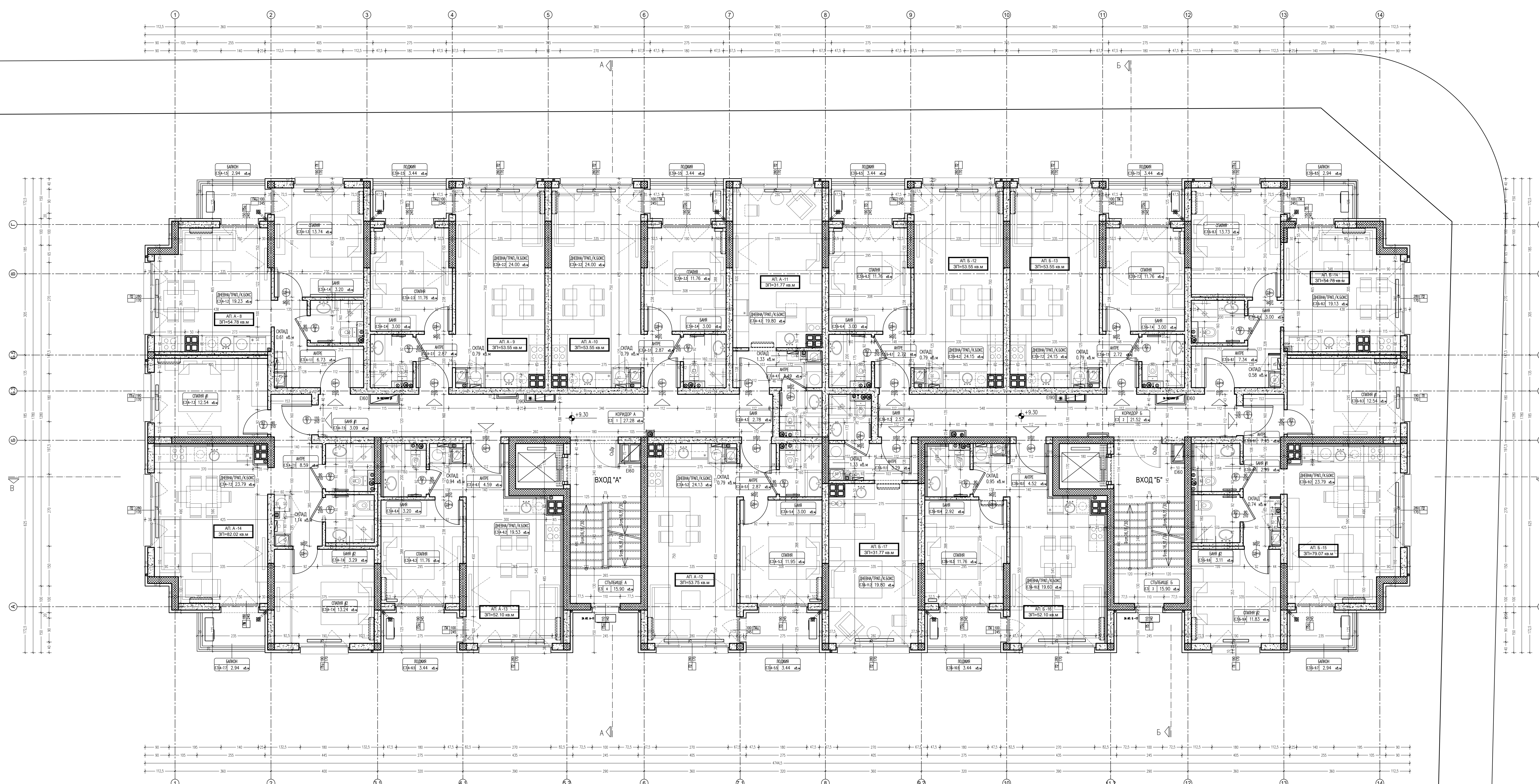
ПЛАН НА КОТА +9.30 /ЕТАЖ 3/ М 1:50
